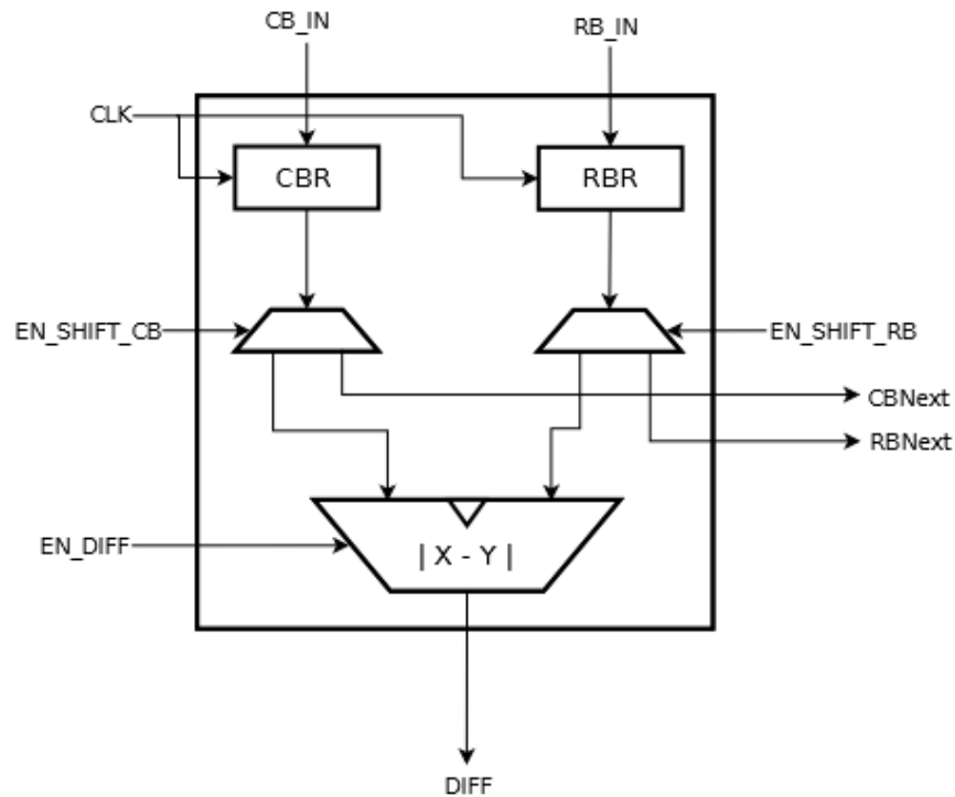
Σχήμα 3.4: Ένα Στοιχείο Επεξεργασίας (Processing Element)
