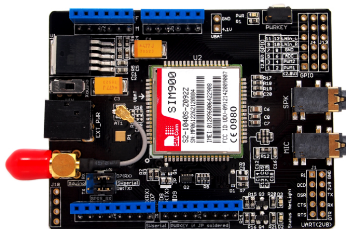
Σχήμα 4.2: GPRS shield
