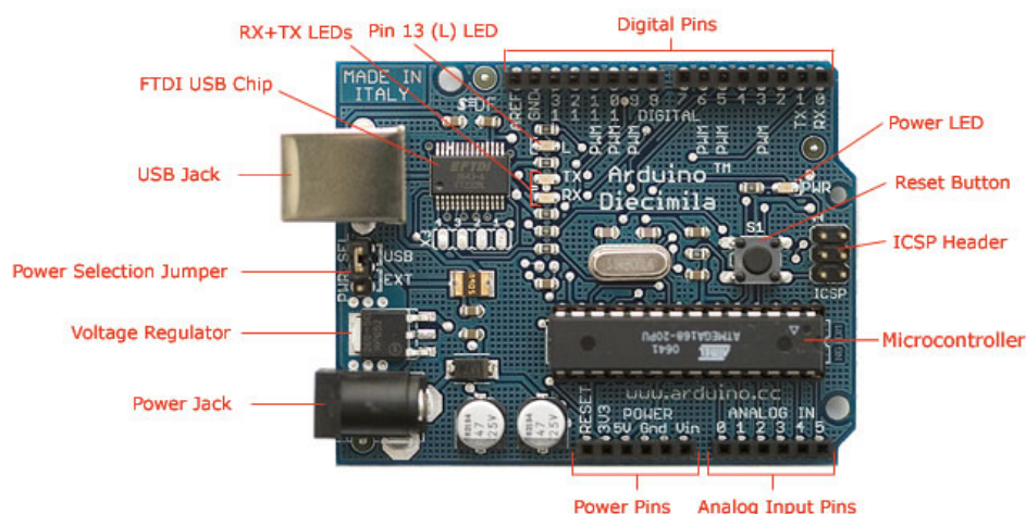
Σχήμα 4.1: Arduino Diecimila
