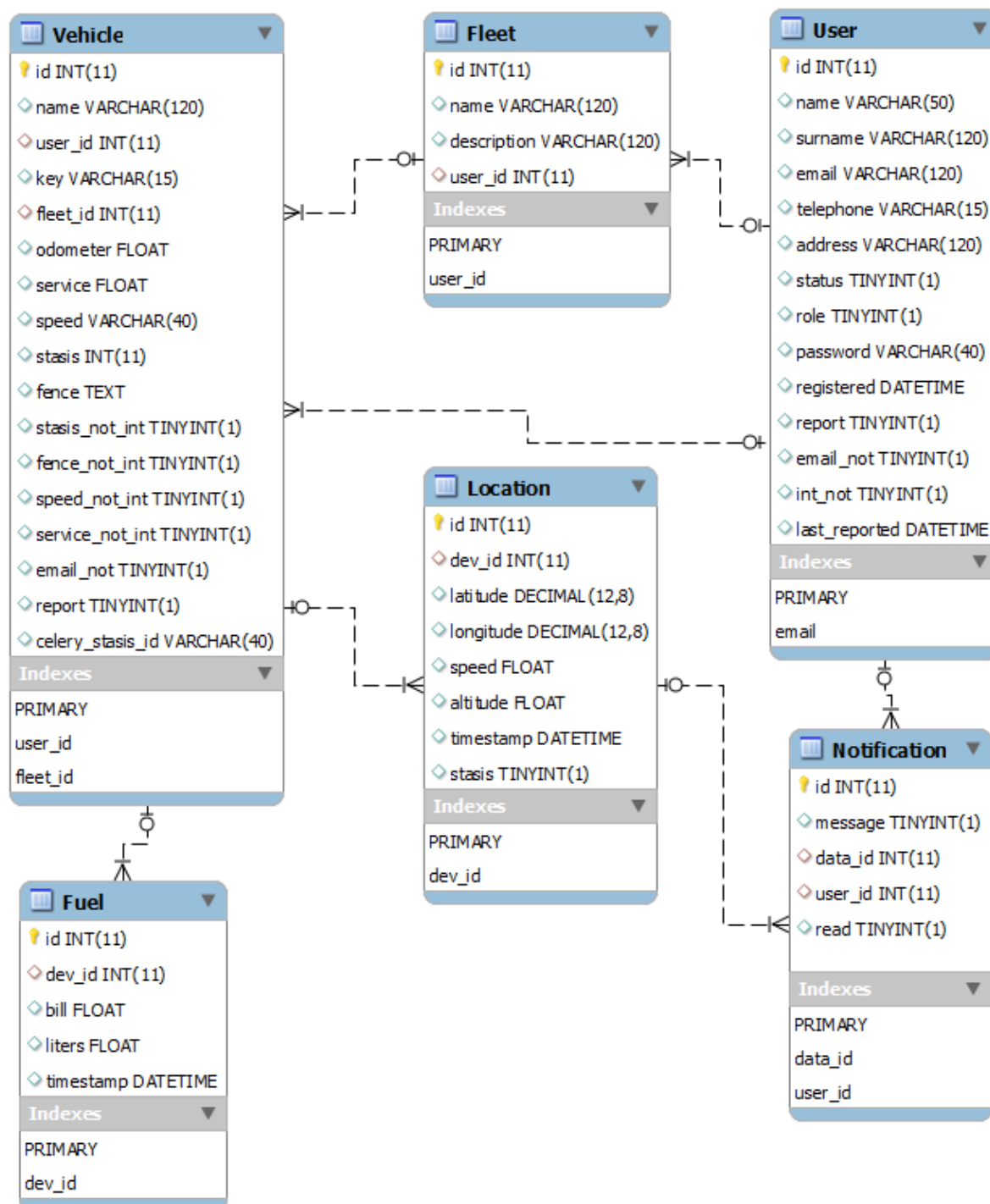
Σχήμα 2.3: Διάγραμμα οντοτήτων-συσχετίσεων
