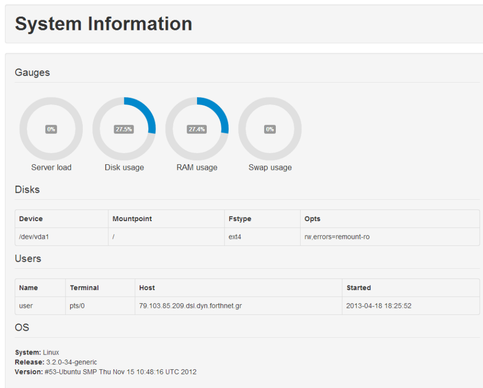
Σχήμα 3.26: Πληροφορίες συστήματος
